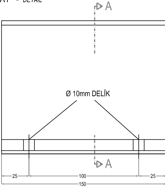
Görünüş
