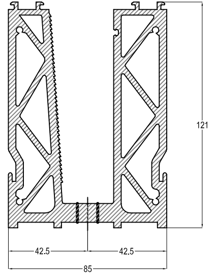
A - A KESİTİ
