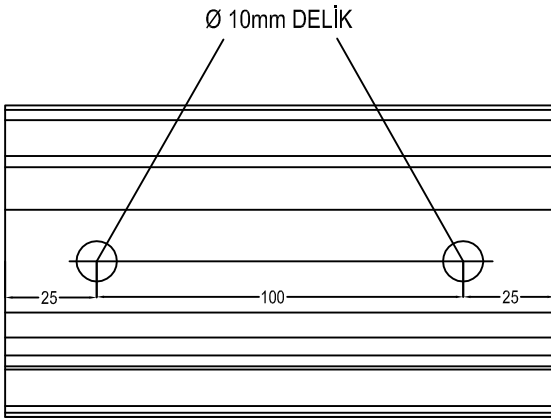
Üst Görünüş
